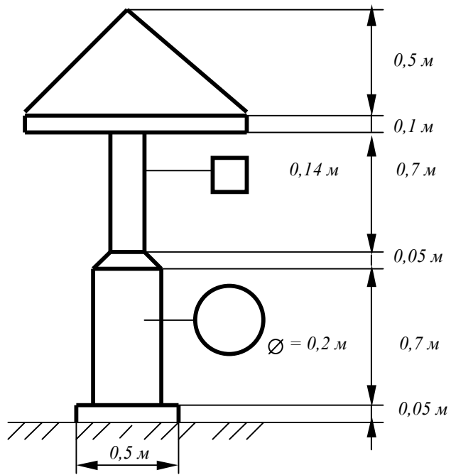
План крыши гриба
